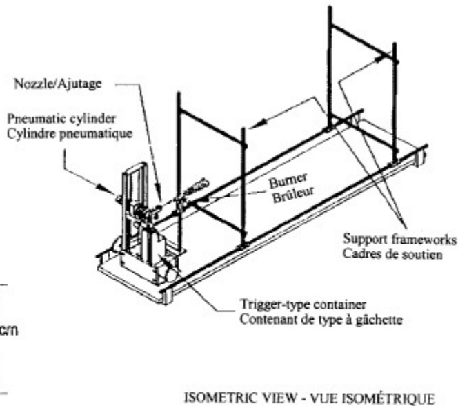
FIGURE 2 Dispositif vérificateur d'inflammabilité Atomiseur
