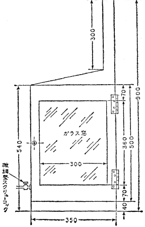
[その4] 正面 (単位 ミリメートル)
