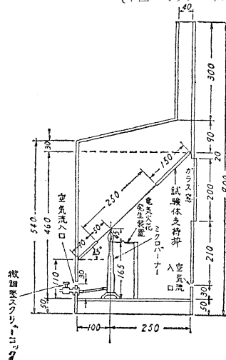
別図第1 燃焼試験箱(第4条の3関係)
