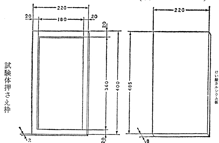
別図第2の3 試験体押さえ枠及びけい酸カルシウム板(第4条の3関係)
