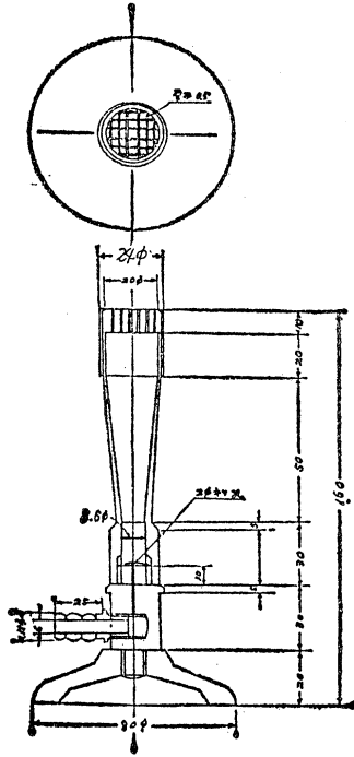
別図第5 メッケルバーナー(第4条の3関係) (単位 ミリメートル)
