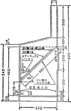
[その3] (じゅうたん等の場合) (単位 ミリメートル)
