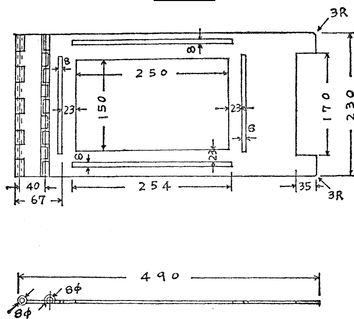
(その2)(単位ミリメートル)
