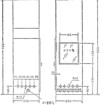
[その5] 側面 (単位 ミリメートル)
