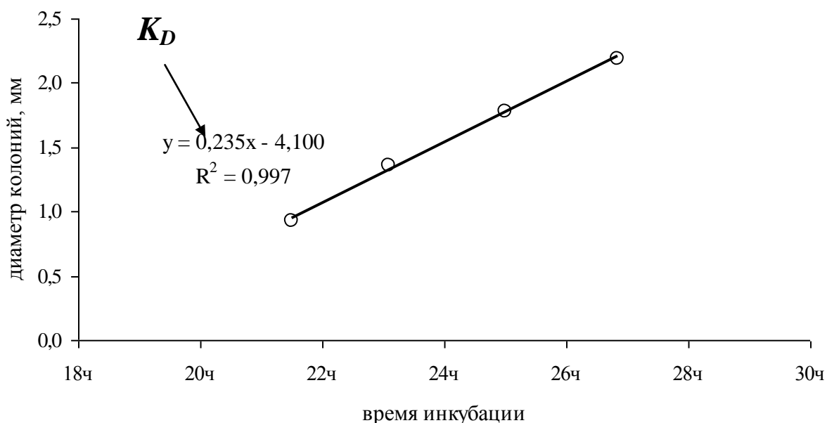
Рисунок 1. Пример определения значения показателя K_D для роста колоний Ps. fluorescens ATCC 27663 на ГРМ-агаре.
