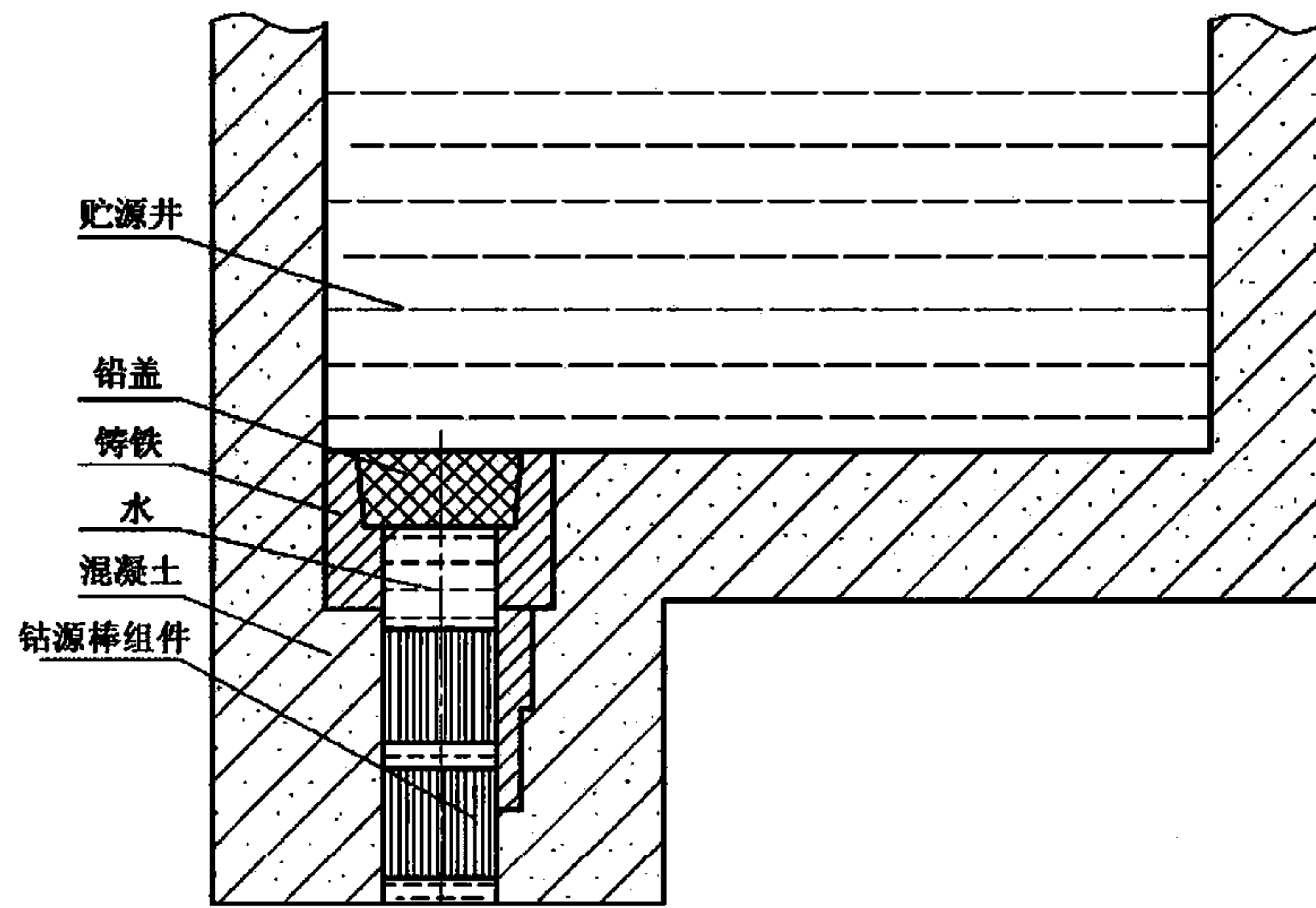
图 A.5 副井屏蔽计算图
