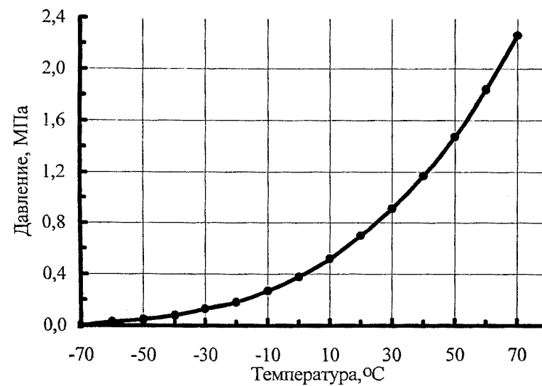
Равновесное давление (абсолютное) насыщенных паров хлора над жидкостью в закрытом сосуде
