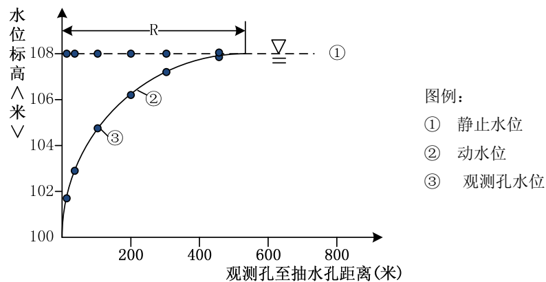
图 C.1 图解法确定影响半径示意图
