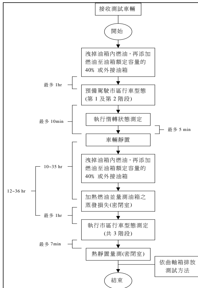
圖一 火花點火引擎車輛排放污染及蒸發排放測試步驟
